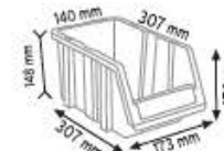
P.A 315 x 30 adet
