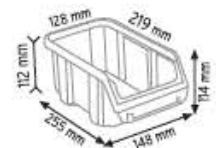
A200 x 28 adet
