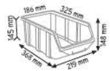
A300 x 8 adet
